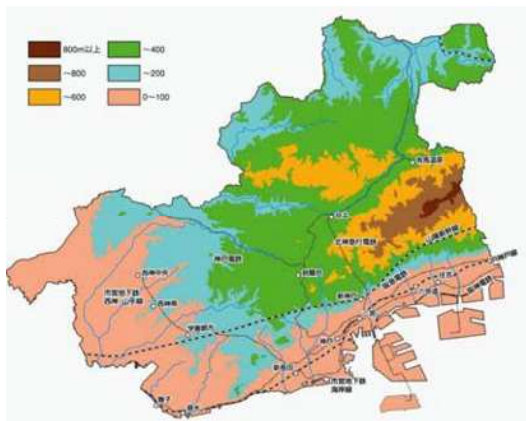
図2-1 神戸の標高
