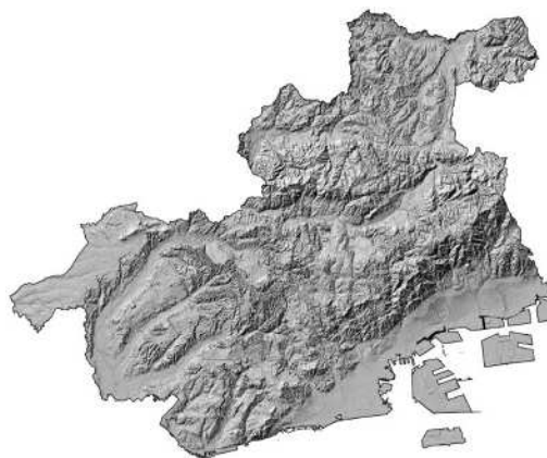
図2-2 神戸の起伏
