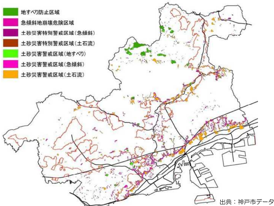
図 2-41 土砂災害等危険区域指定状況
