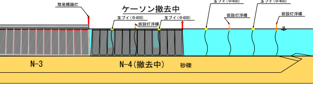
仮設標識灯および仮設灯浮標設置概要図
