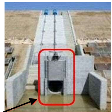
取水部(斜樋)
