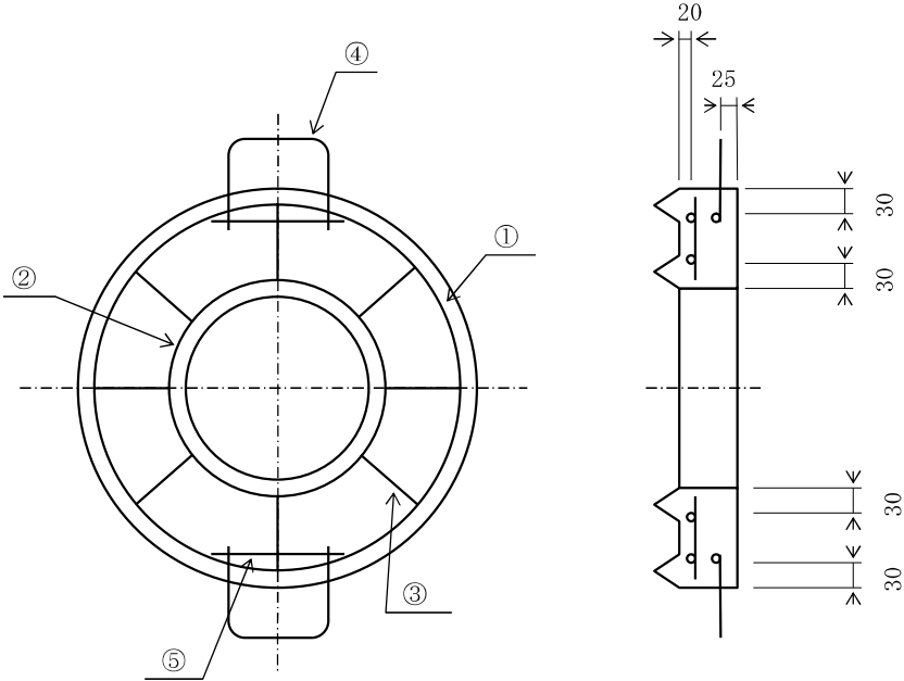
4), 仕切弁基礎ブロック 250 配筋図 (A 型)
