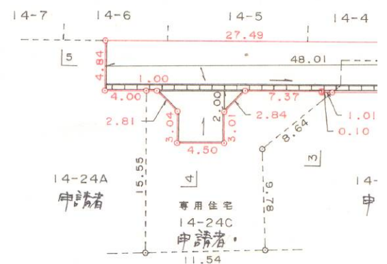
道路平面図 S =
