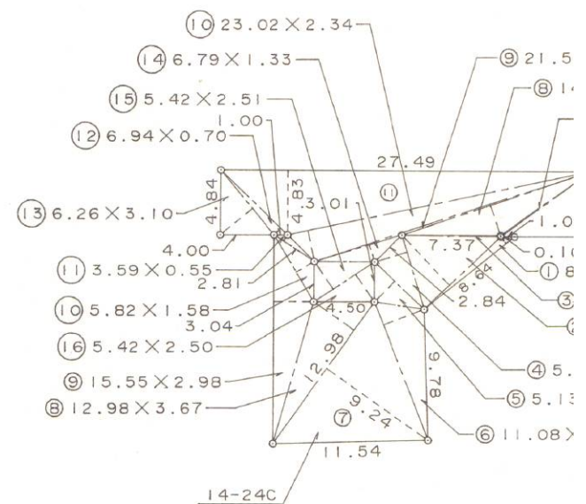
敷地求積図 S =
