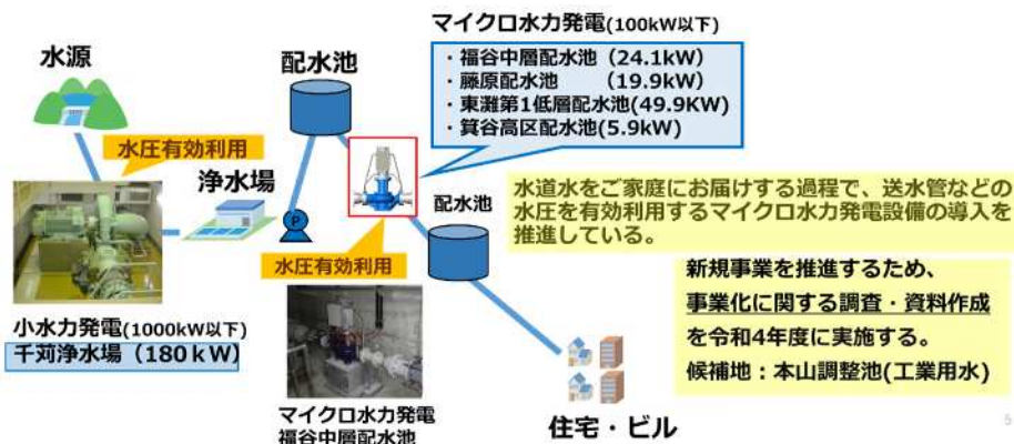
図 21 神戸の水道施設を活用した水力発電
