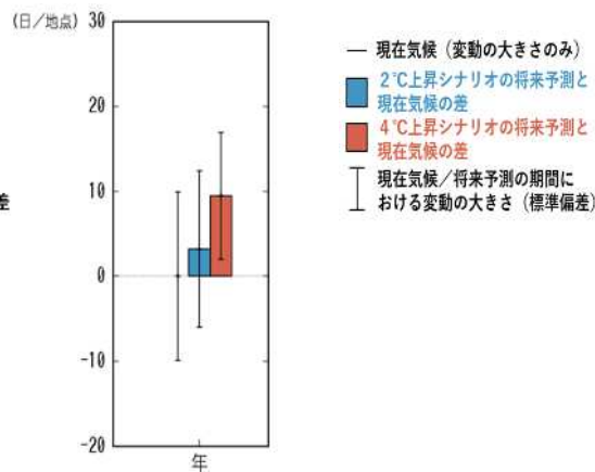
図 38 無降水日数の変化
