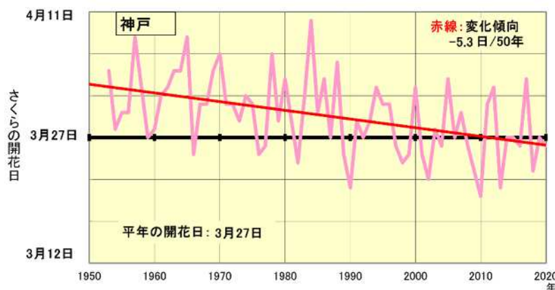
図 34 神戸のさくらの開花日
