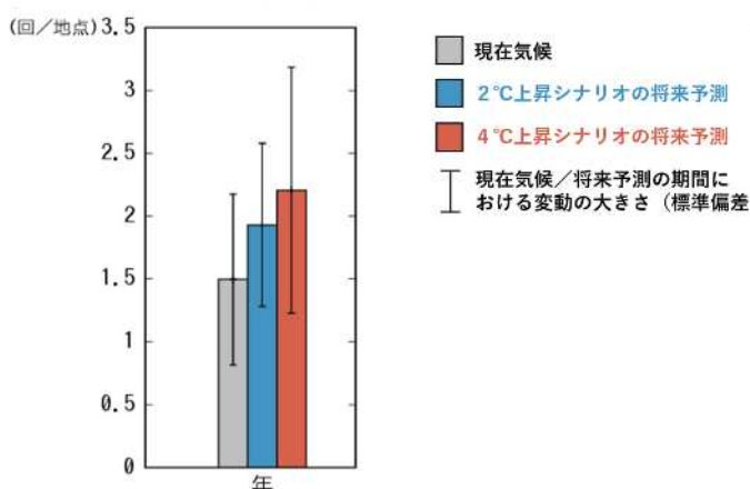
図 37 1時間降水量30mm以上の発生回数の変化
