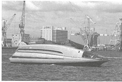
超電導電磁推進船「ヤマト1」(280 G/T)
