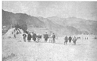
生田川付替工事
