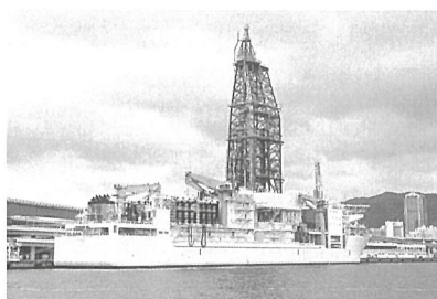
「ちきゅう」(57,087 G/T)
