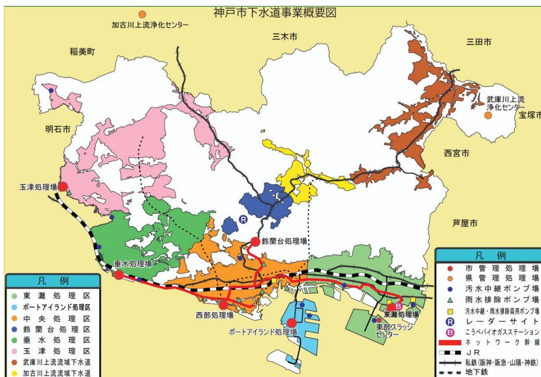
■下水道処理施設の配置図
