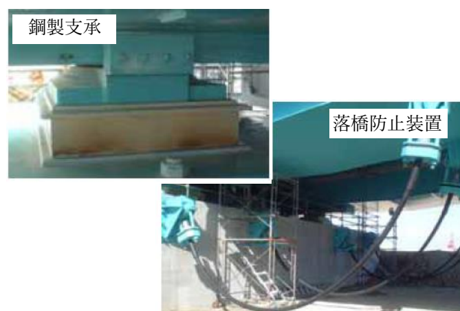
図 22 空港連絡橋における耐震対策
