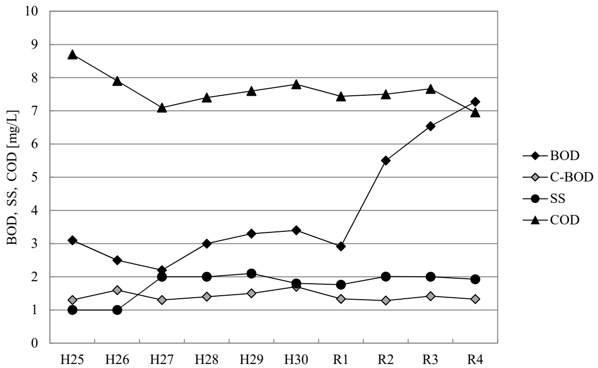
(3)放流水質(加重平均)
