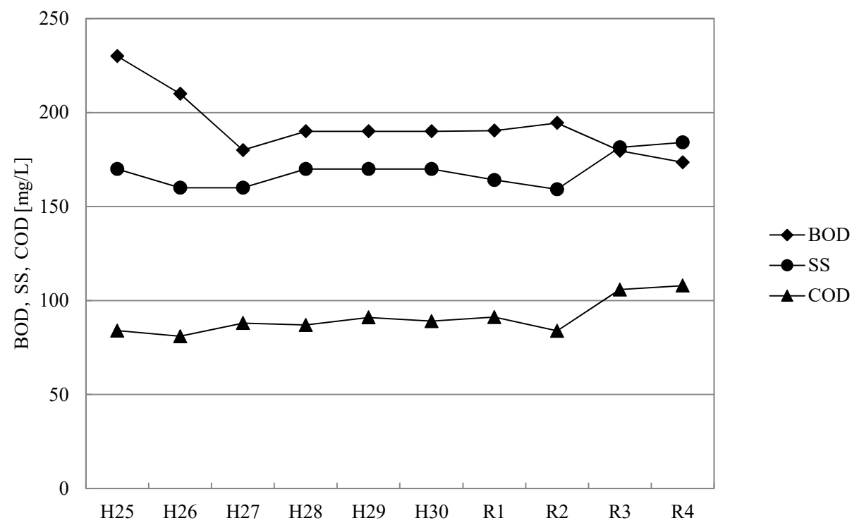
(2) 流入水質(加重平均)
