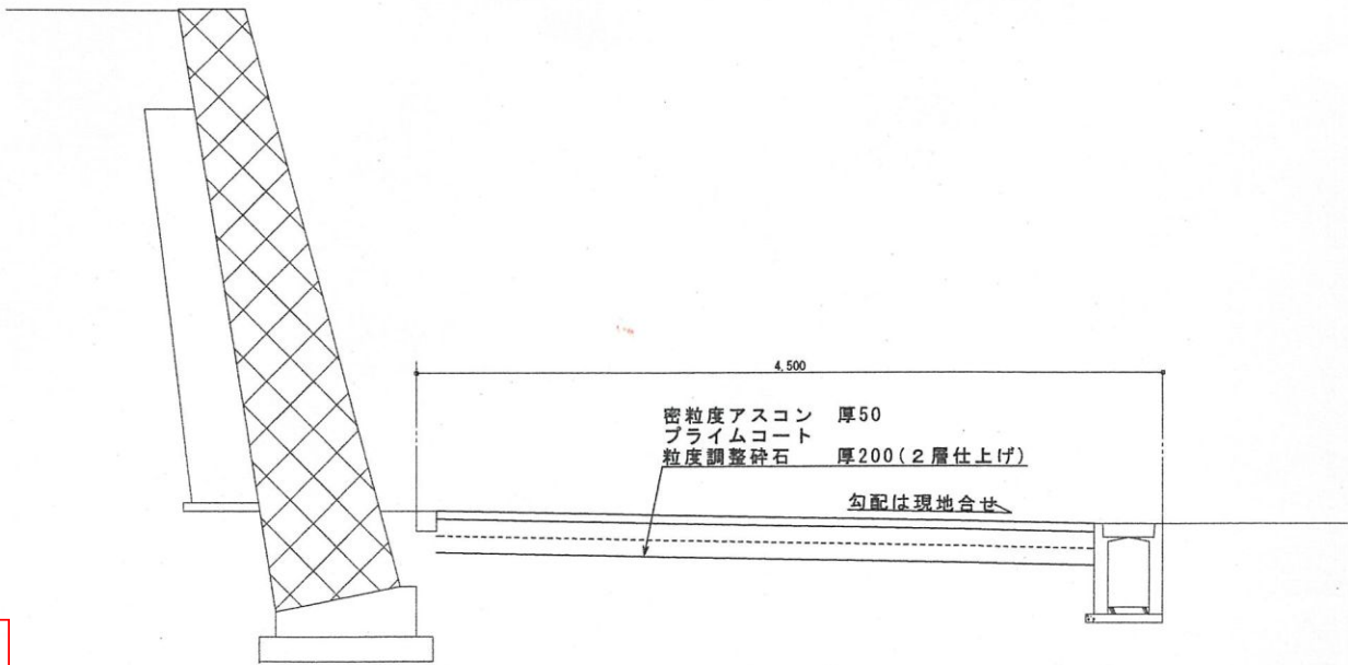
断面図 S:1/50
