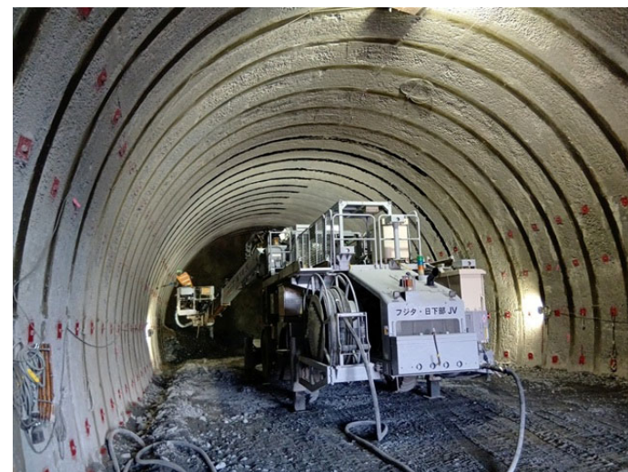
④ 支保工二次吹付コンクリート施工状況
